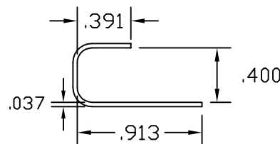
P/N 138
