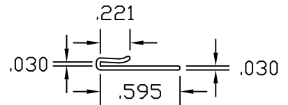
P/N 891
