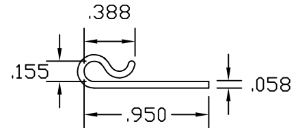
P/N 290
