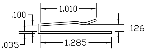
P/N 196
