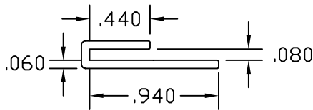
P/N 907
