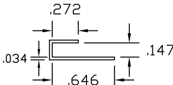
P/N 148
