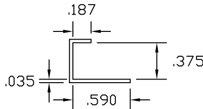
P/N 360
